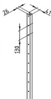
profil metalic de fixare pe stalp de 25, tip U prevazut cu gauri
