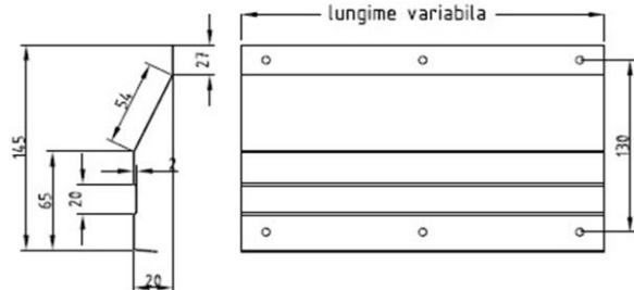
lamela orizontala X 135
