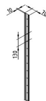
rigla metalica de rigidizare
