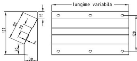
lamela orizontala X 121
