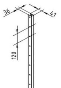
profil metalic de fixare pe stalp de 35, tip U, prevazut cu gauri
