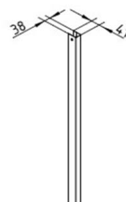
capac inchidere gard, tip U (stalp de 35)
